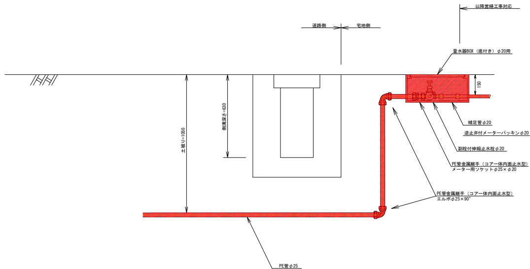
給水装置標準図 S=1/10
