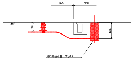
A部断面図
